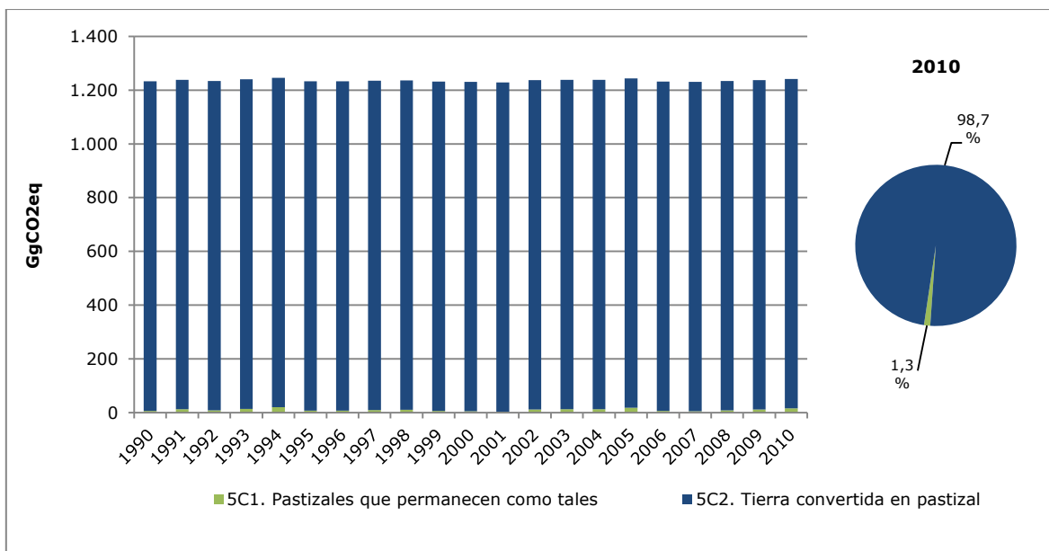
Figura 66. Pastizales: tendencia de las emisiones y absorciones de GEI por subcategoría, serie 1990-2010
