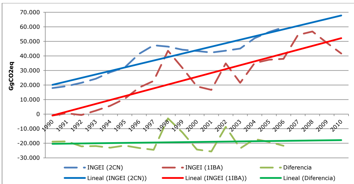
Figura 78. INGEI de Chile: tendencia de las emisiones netas de GEI reportadas por Chile en la Segunda Comunicación Nacional y en el Primer Informe Bienal de Actualización, serie 1990-2010
