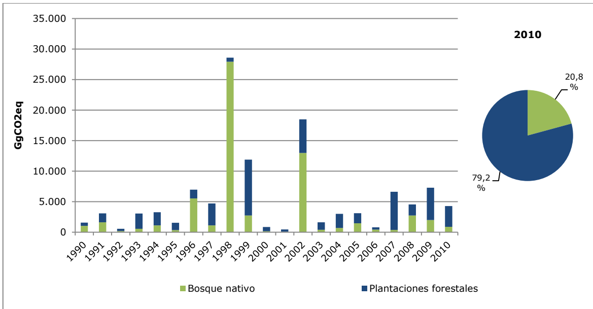
Figura 58. Incendios forestales: emisiones de GEI por incendios en bosque nativo y plantaciones forestales, serie 1990-2010
