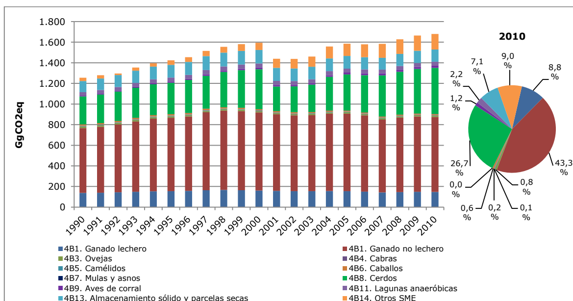
Figura 44. Manejo del estiércol: tendencia de las emisiones de GEI por especie y sistema de manejo del estiércol, serie 1990-2010
