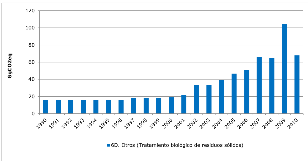
Figura 77. Otros (Tratamiento biológico de residuos sólidos): tendencia de las emisiones de GEI, serie 1990-2010
