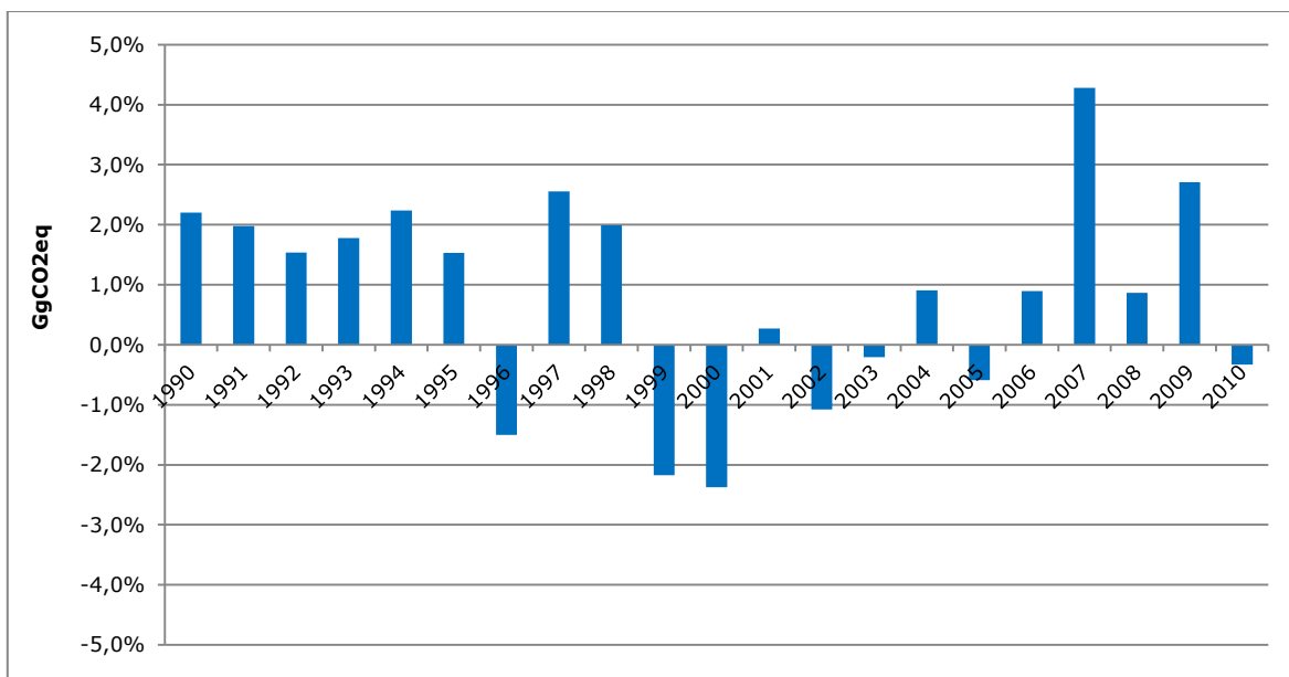
Figura 25. Quema de combustible: diferencia porcentual entre el método sectorial y el método de referencia, serie 1990-2010
