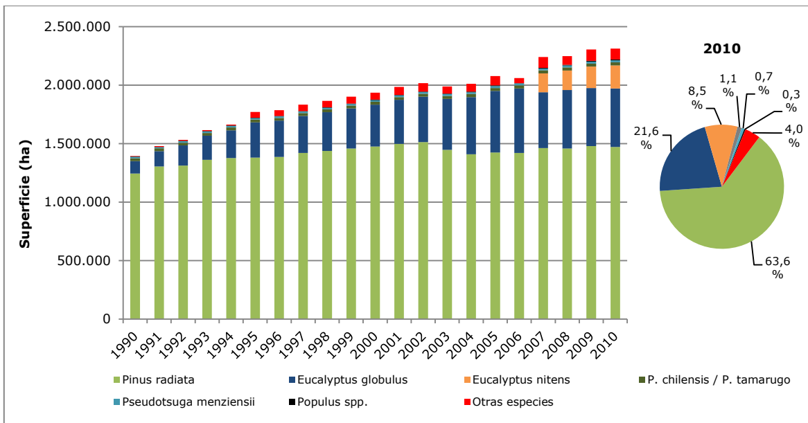
Figura 62. Plantaciones forestales: tendencia de la superficie anual por especie, serie 1990-2010
