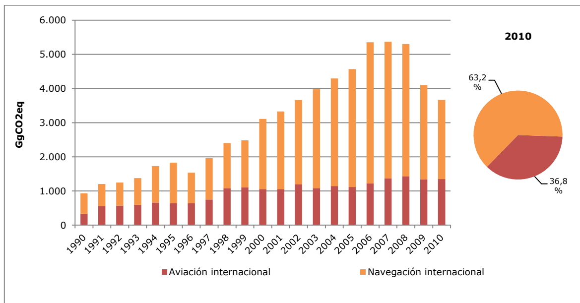
Figura 26. Búnker internacional: tendencia de las emisiones de GEI por tipo de transporte internacional, serie 1990-2010
