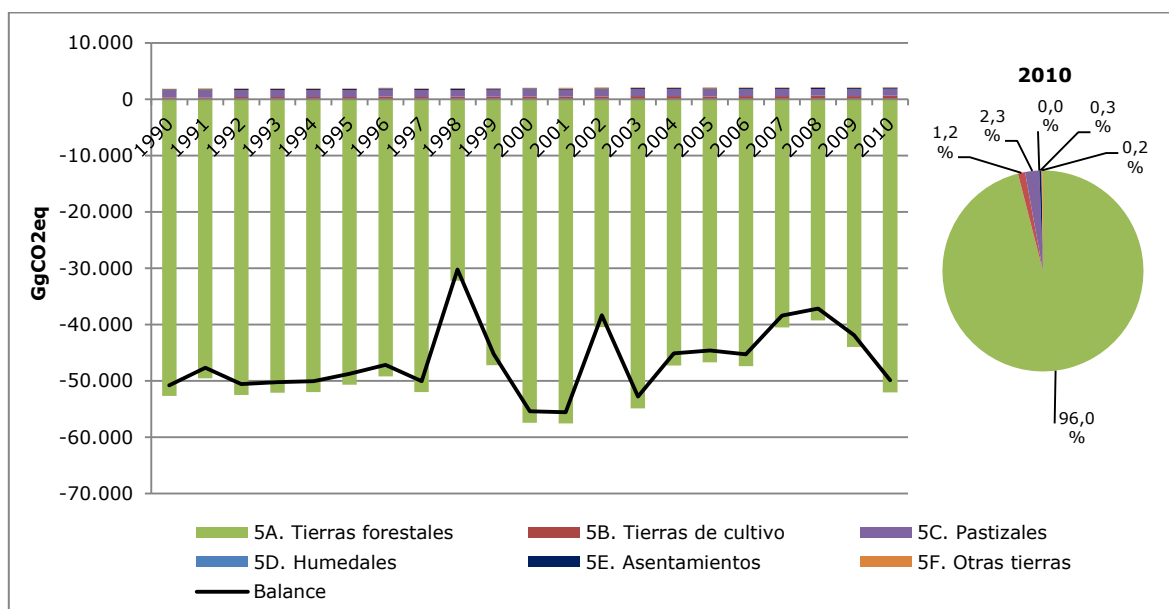
Figura 50. Sector UTCUTS: tendencia de las emisiones y absorciones de GEI por categoría, serie 1990-2010
