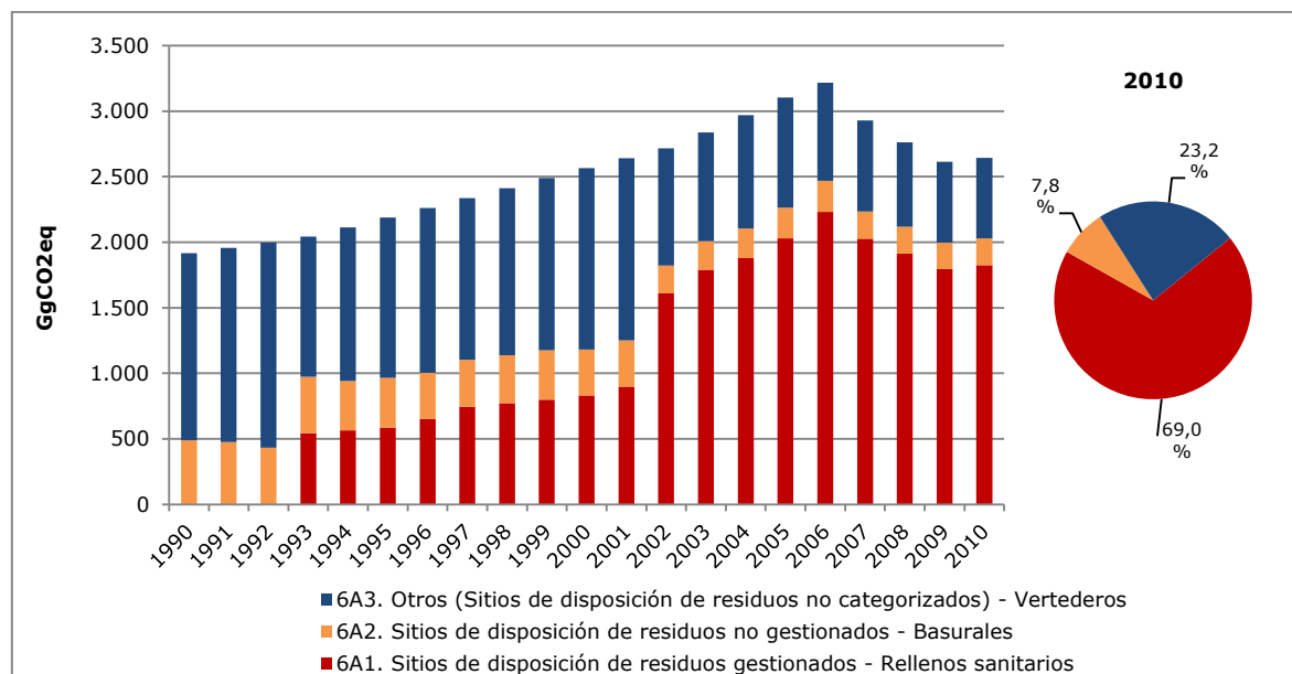
Figura 72. Disposición de residuos sólidos: tendencia de las emisiones de GEI por subcategoría, serie 1990-2010
