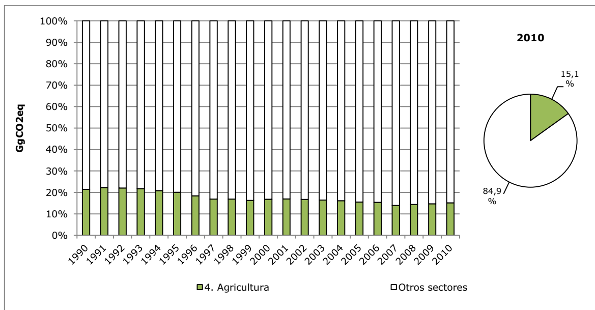
Figura 38. Sector Agricultura: tendencia de la participación del sector en las emisiones de GEI totales (excl. UTCUTS)
