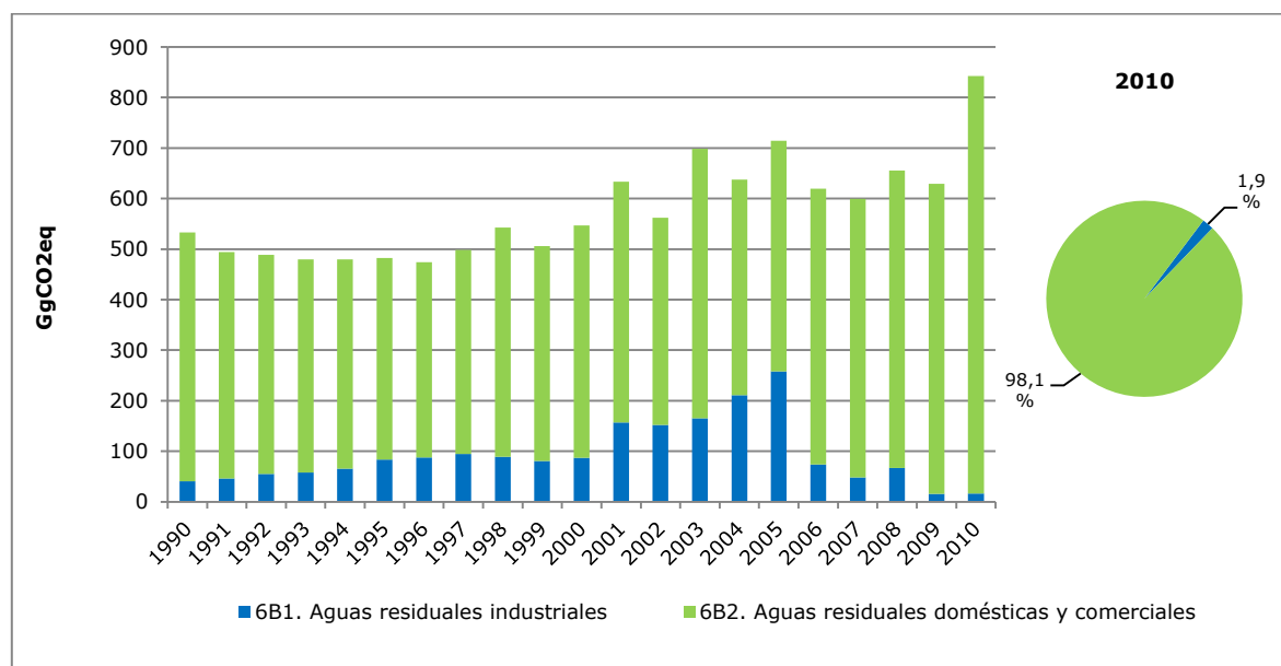
Figura 75. Tratamiento y descarga de aguas residuales: tendencia de las emisiones de GEI por subcategoría, serie 1990-2010
