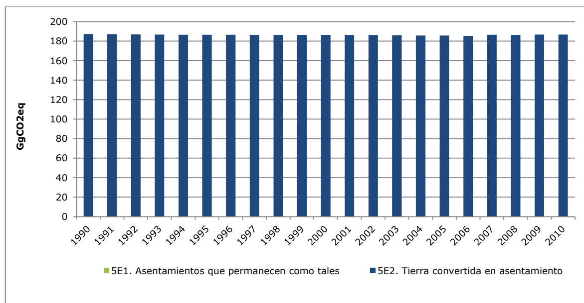
Figura 67. Asentamientos: tendencia de las emisiones y absorciones de GEI por subcategoría, serie 1990-2010
