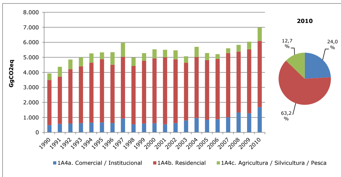
Figura 21. Otros sectores: tendencia de las emisiones de GEI por componente, serie 1990-2010
