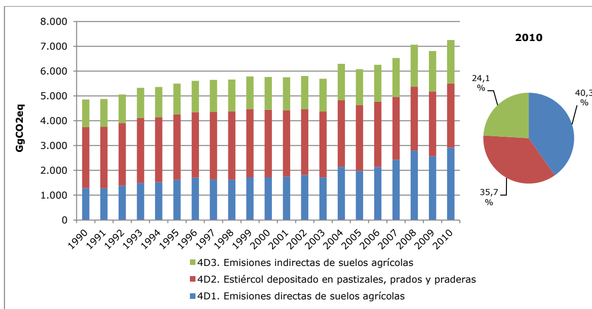
Figura 46. Suelos agrícolas: tendencia de las emisiones de GEI por subcategoría, serie 1990-2010
