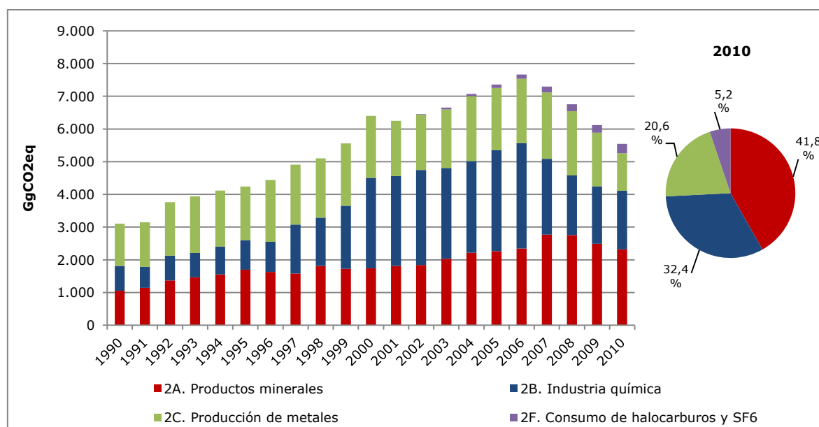
Figura 29. Sector Procesos industriales: tendencia de las emisiones de GEI por categoría, serie 1990-2010
