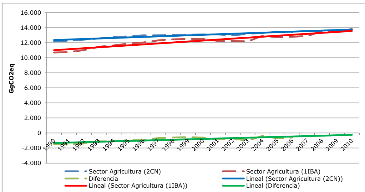
Figura 81. Sector Agricultura: tendencia de las emisiones de GEI reportadas por Chile en la Segunda Comunicación Nacional y en el Primer Informe Bienal de Actualización, serie 1990-2010
