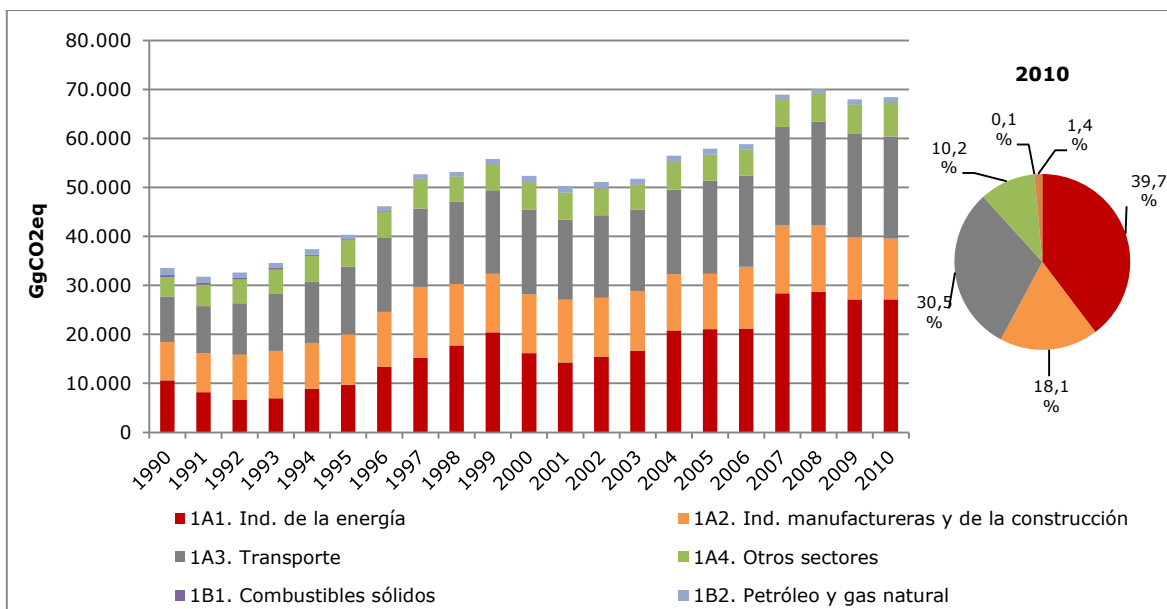
Figura 10. Sector Energía: tendencia de las emisiones de GEI por subcategoría, serie 1990-2010
