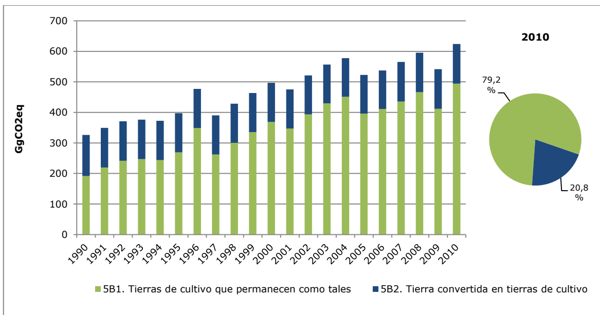
Figura 65. Tierras de cultivo: tendencia de las emisiones y absorciones de GEI (GgCO 2 eq) por subcategoría, serie 1990-2010
