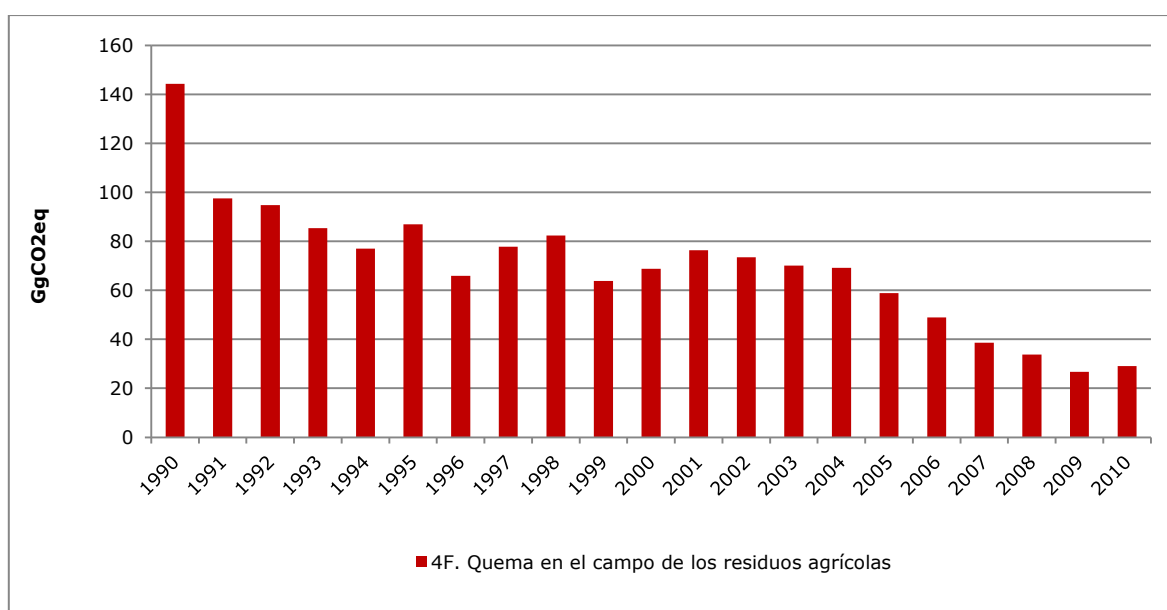
Figura 49. Quema en el campo de los residuos agrícolas: tendencia de las emisiones de GEI, serie 1990-2010
