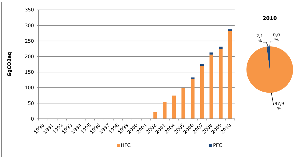
Figura 6. INGEI de Chile: tendencia de las emisiones de gases fluorados por tipo de GEI y excluyendo UTCUTS, serie 1990-2010
