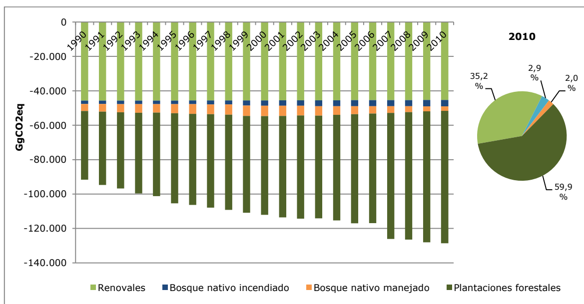
Figura 55. Incremento en biomasa: tendencia de las absorciones de CO 2 por componente, serie 1990-2010
