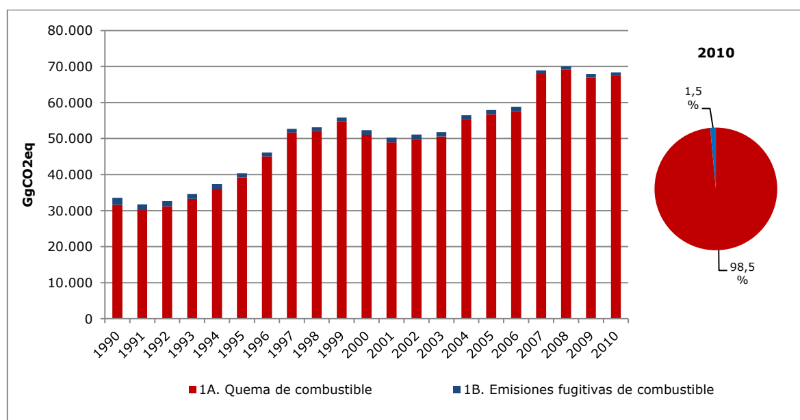
Figura 9. Sector Energía: tendencia de las emisiones de GEI por categoría, serie 1990-2010
