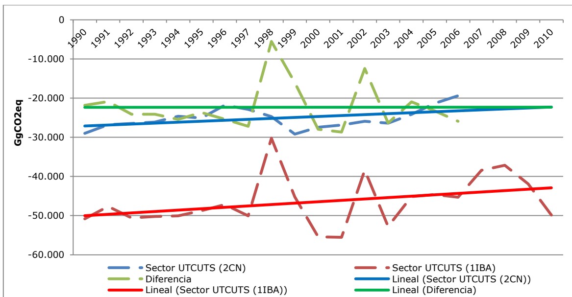
Figura 82. Sector UTCUTS: tendencia de las emisiones netas de GEI reportadas por Chile en la Segunda Comunicación Nacional y en el Primer Informe Bienal de Actualización, serie 1990-2010
