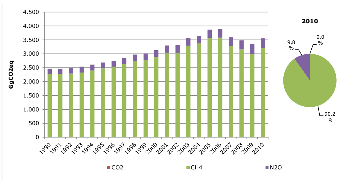
Figura 71. Sector Residuos: tendencia de las emisiones por tipo de GEI, serie 1990-2010
