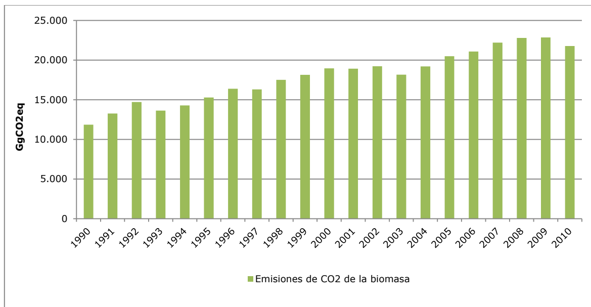
Figura 27. Emisiones de CO 2 de la biomasa: tendencia de las emisiones de CO 2 , serie 1990-2010
