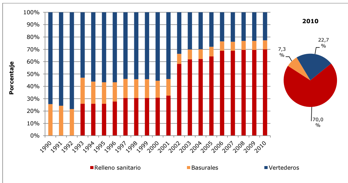
Figura 74. Disposición de residuos sólidos: tendencia de la fracción de residuos sólidos domiciliarios por sitio de disposición final, serie 1990-2010
