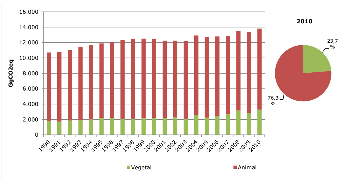
Figura 41. Sector Agricultura: tendencia de las emisiones de GEI de origen vegetal y origen animal, serie 1990-2010
