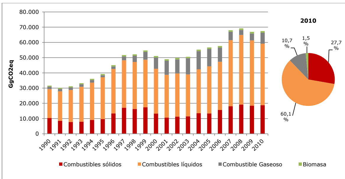
Figura 13. Quema de combustible: emisiones de GEI (GgCO 2 eq) por tipo de combustible, serie 1990-2010
