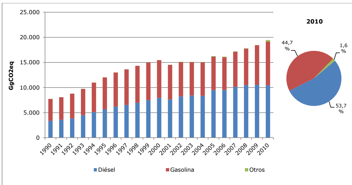
Figura 20. Transporte terrestre: tendencia de las emisiones de GEI por combustible, serie 1990-2010
