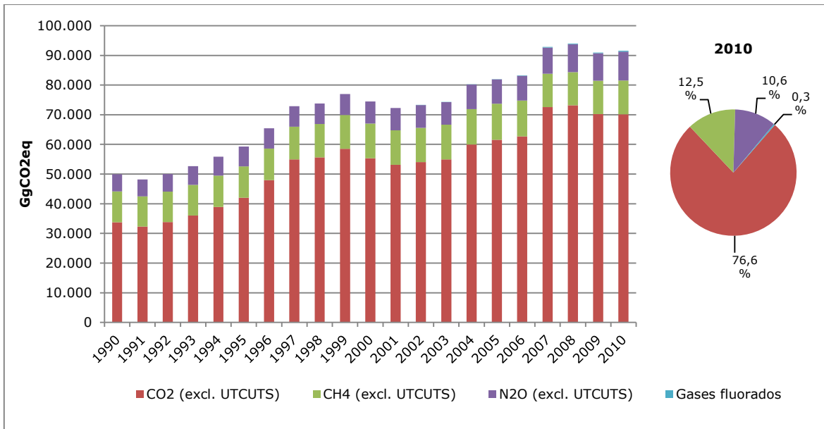
Figura 5. INGEI de Chile: tendencia de las emisiones de GEI por tipo de GEI y excluyendo UTCUTS, serie 1990-2010
