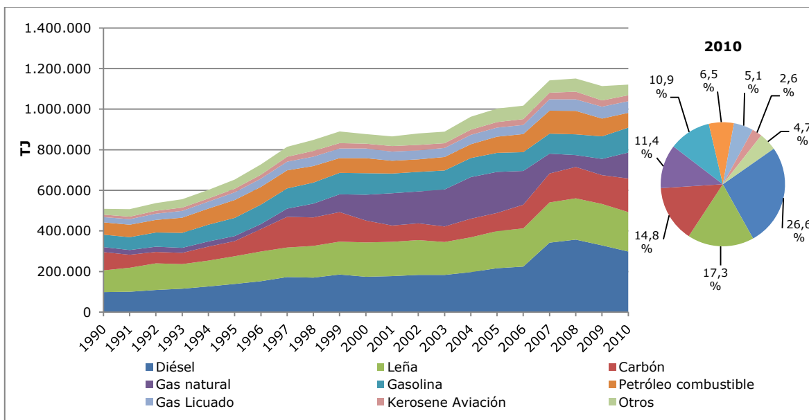
Figura 7. Sector Energía: tendencia del consumo de combustibles (TJ) por tipo de combustible, serie 1990-2010
