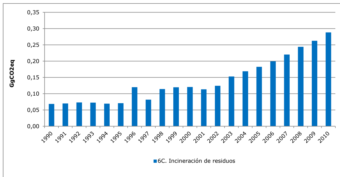
Figura 76. Incineración de residuos: tendencia de las emisiones de GEI, serie 1990-2010
