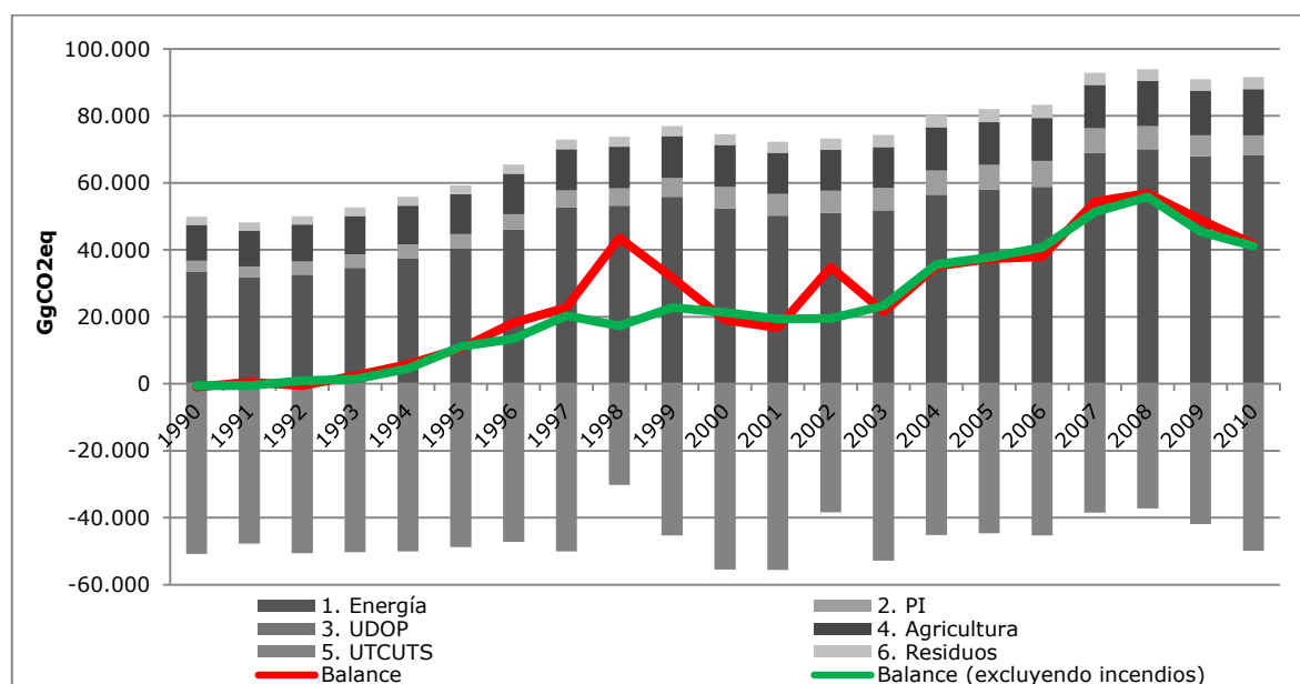
Figura 60. INGEI de Chile: tendencia de las emisiones y absorciones de GEI por sector excluyendo incendios en bosques, serie 1990-2010
