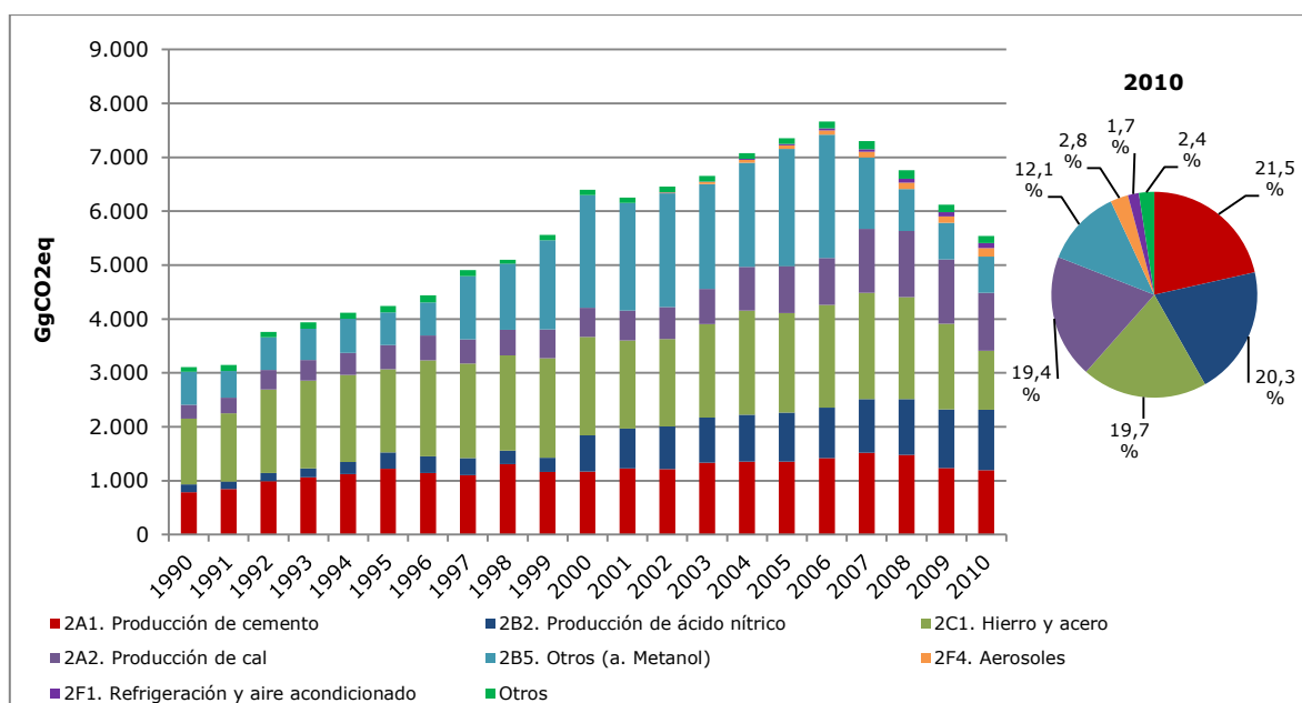
Figura 30. Sector Procesos industriales: tendencia de las emisiones de GEI por subcategoría, serie 1990-2010
