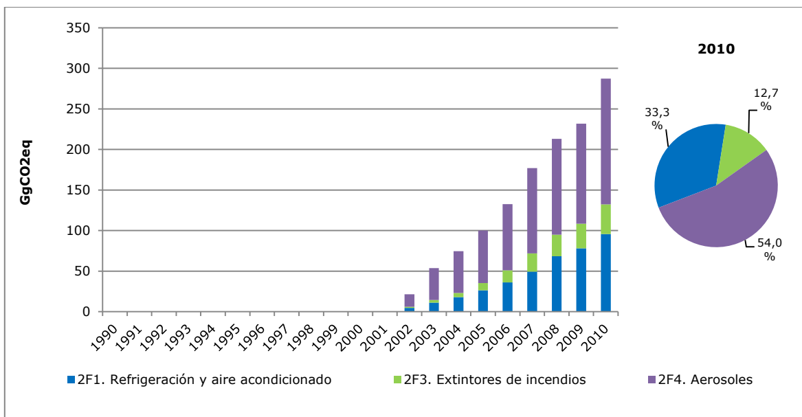
Figura 35. Consumo de halocarburos y SF 6 : tendencia de las emisiones de GEI por subcategoría, serie 1990-2010
