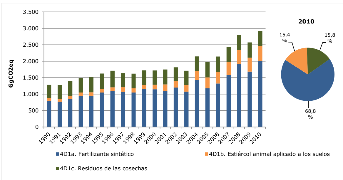
Figura 47. Emisiones directas de suelos agrícolas: tendencia de las emisiones de GEI por componente, serie 1990-2010
