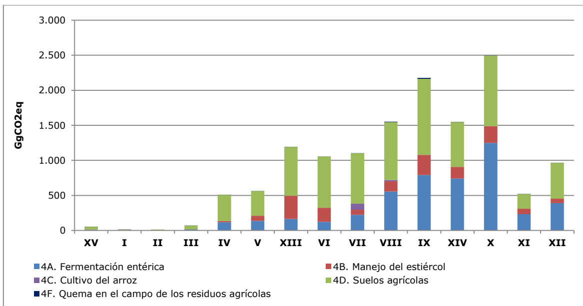
Figura 42. Sector Agricultura: emisiones de GEI por categoría y región administrativa, año 2010
