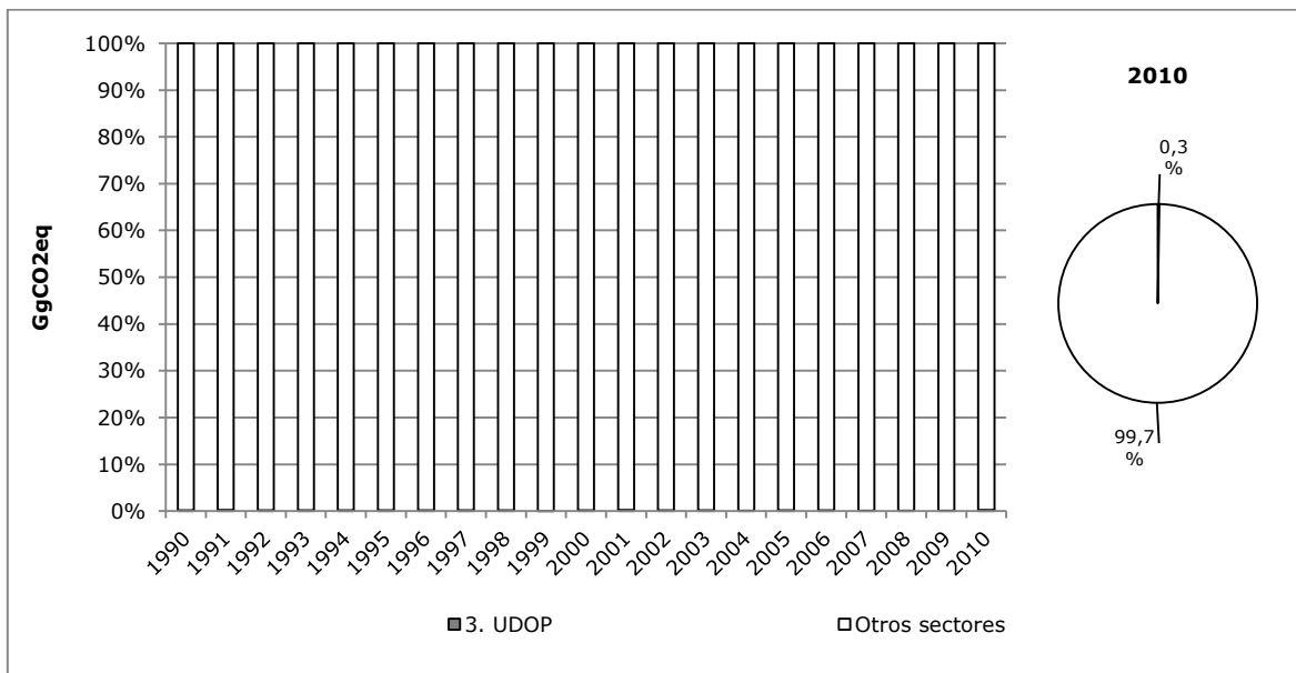
Figura 36. Sector UDOP: tendencia de la participación del sector en las emisiones de GEI totales (excl. UTCUTS)
