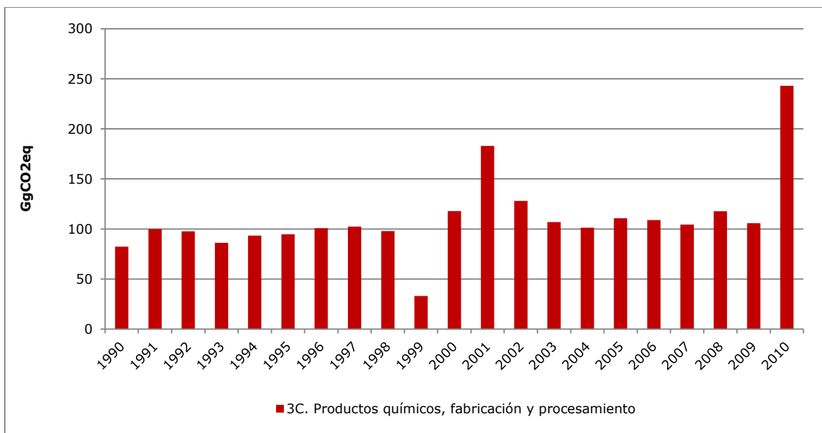
Figura 37. Sector UDOP: tendencia de las emisiones de GEI por categoría, serie 1990-2010
