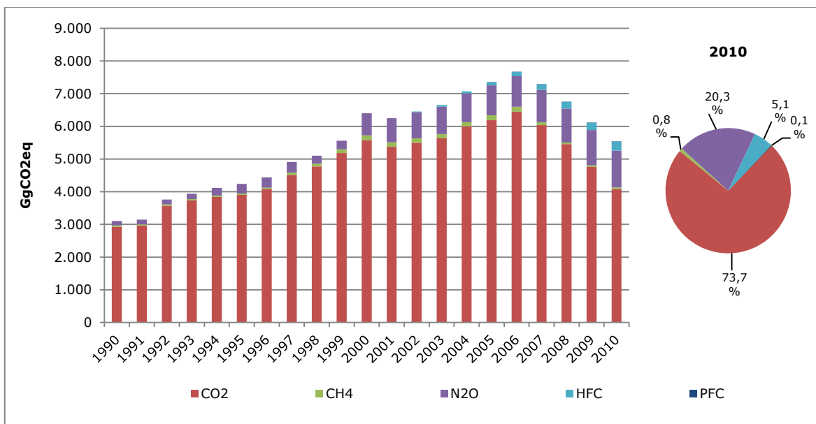
Figura 31. Sector Procesos industriales: emisiones por tipo de GEI (GgCO 2 eq), serie 1990-2010
