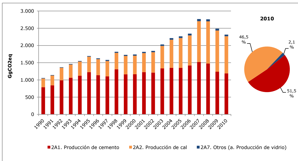
Figura 32. Productos minerales: tendencia de las emisiones de GEI por subcategoría, serie 1990-2010
