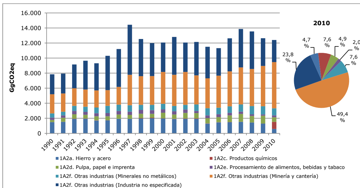
Figura 17. Industrias manufactureras y de la construcción: tendencia de las emisiones de GEI por componente, serie 1990-2010
