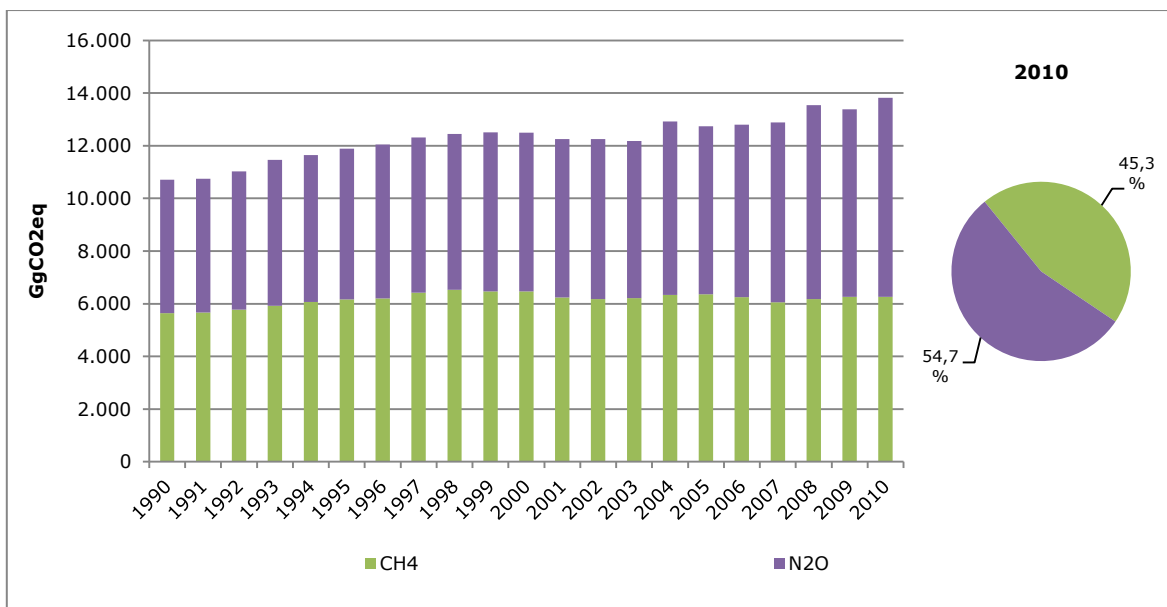
Figura 40. Sector Agricultura: tendencia de las emisiones por tipo de GEI, serie 1990-2010
