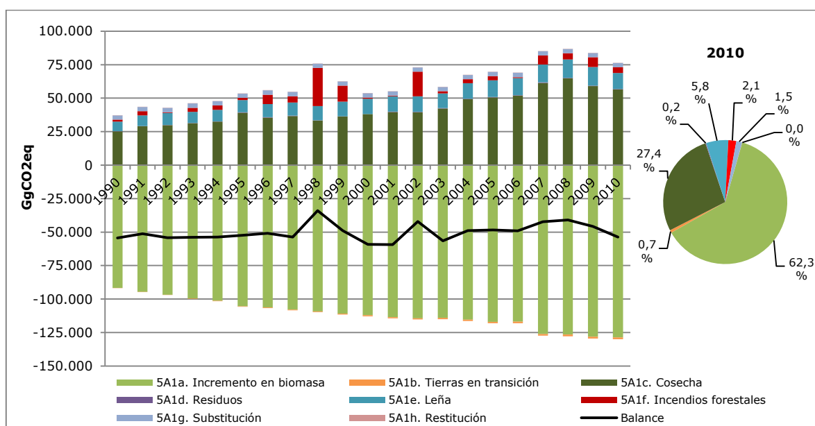
Figura 54. Tierras forestales que permanecen como tales: tendencia de las emisiones y absorciones de GEI por componente, serie 1990-2010
