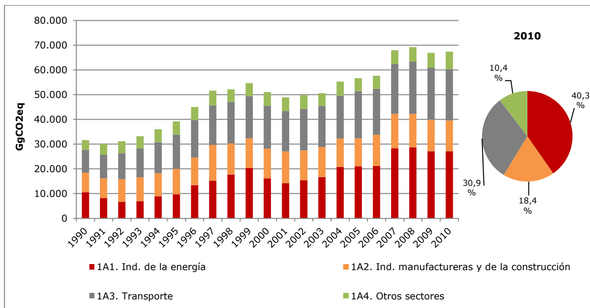
Figura 12. Quema de combustible: tendencia de las emisiones de GEI por subcategoría, serie 1990-2010
