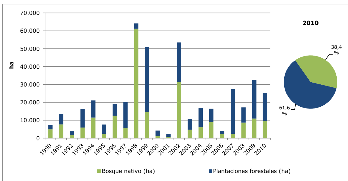
Figura 64. Incendios forestales: tendencia de la superficie anual de bosque nativo y plantaciones forestales afectada por incendios, serie 1990-2010
