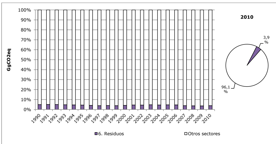
Figura 69. Sector Residuos: tendencia de la participación del sector en las emisiones de GEI totales (excl. UTCUTS)
