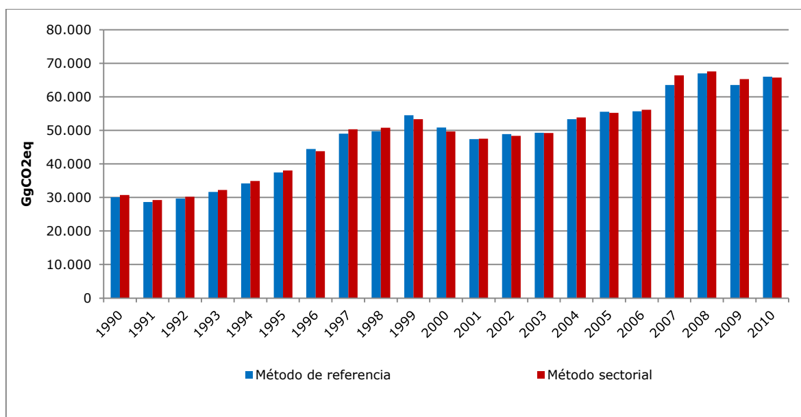
Figura 24. Quema de combustible: emisiones de CO 2 del método sectorial y método de referencia, serie 1990-2010
