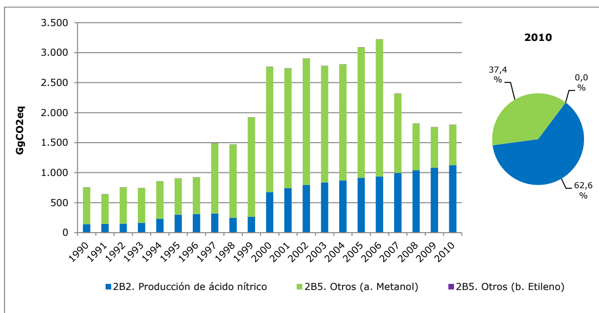
Figura 33. Industria química: tendencia de las emisiones de GEI por subcategoría, serie 1990-2010
