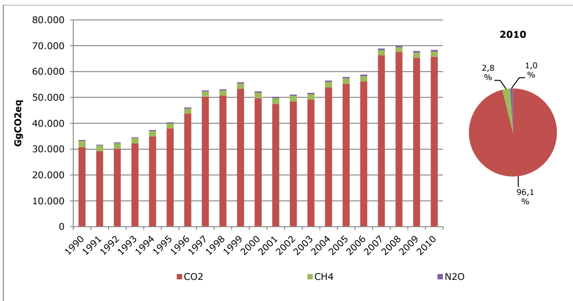
Figura 11. Sector Energía: emisiones por tipo de GEI (GgCO 2 eq), serie 1990-2010
