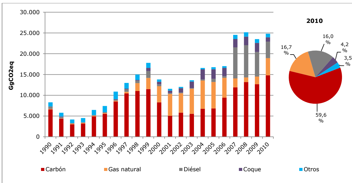
Figura 15. Producción de electricidad y calor como actividad principal: emisiones de GEI (GgCO 2 eq) por combustible, serie 1990-2010
