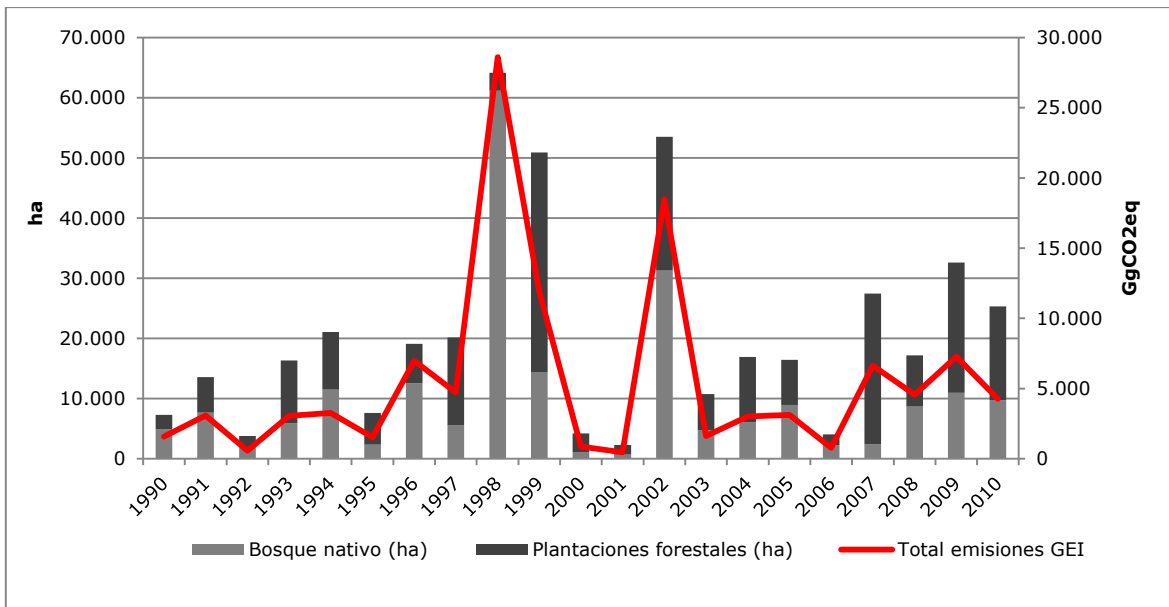
Figura 59. Incendios forestales: tendencia de la superficie anual afectada por incendios y emisiones de GEI, serie 1990-2010
