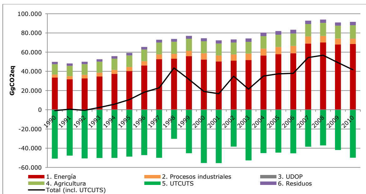
Figura RE.1. INGEI de Chile: tendencia de las emisiones y absorciones de GEI por sector, serie 1990-2010
