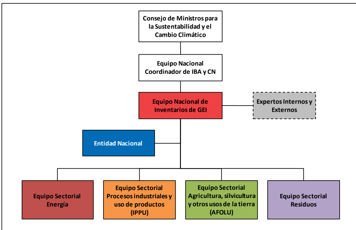
Figura 1. Estructura del Sistema Nacional de Inventarios de GEI de Chile
