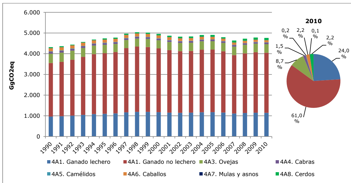
Figura 43. Fermentación entérica: tendencia de las emisiones de GEI por especie, serie 1990-2010
