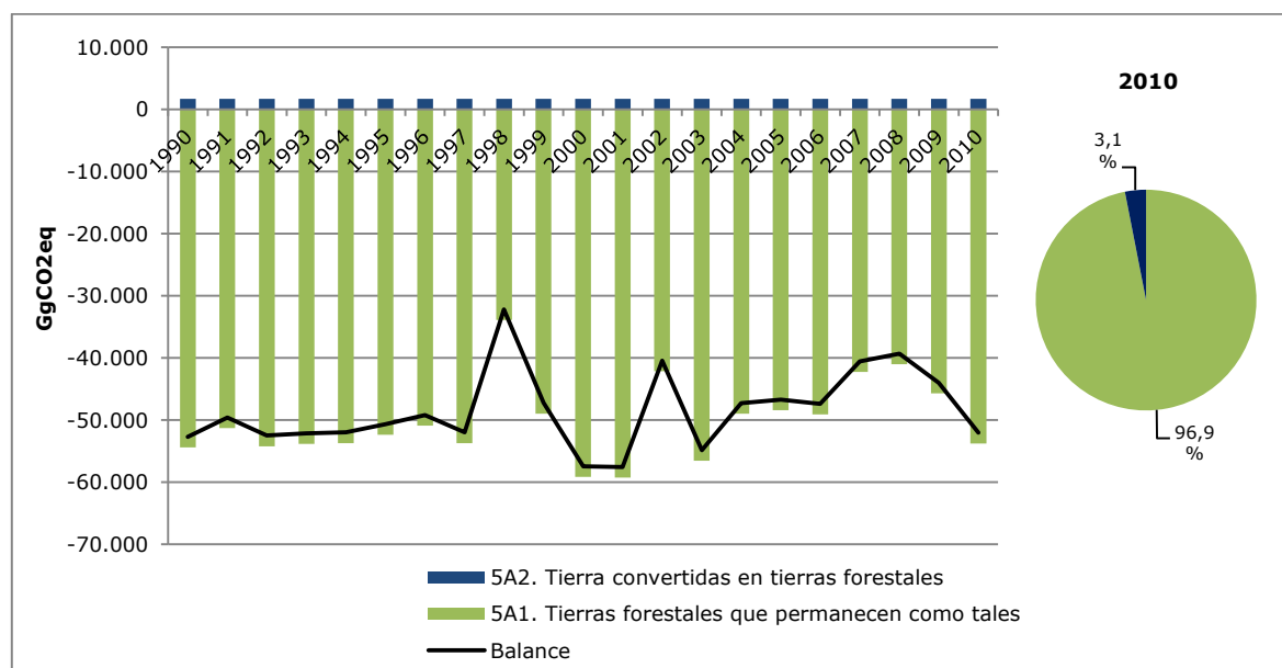
Figura 53. Tierras forestales: tendencia de las emisiones y absorciones de GEI por subcategoría, serie 1990-2010
