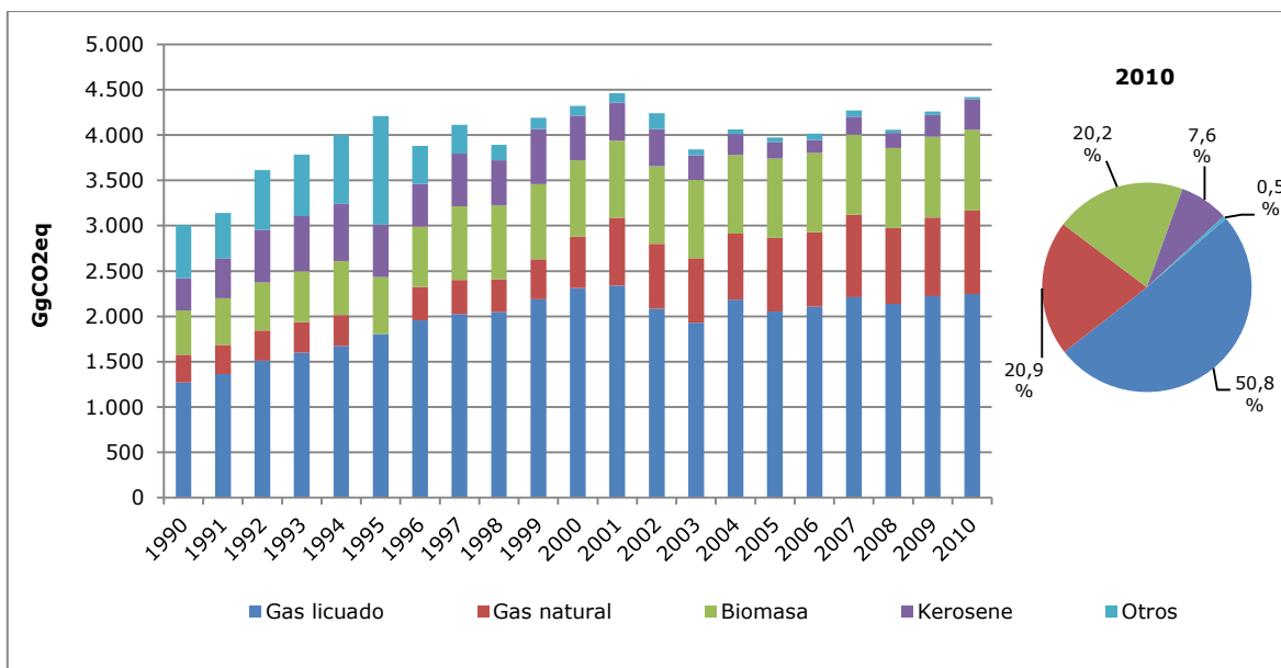
Figura 22. Residencial: tendencia de las emisiones de GEI por combustible, serie 1990-2010
