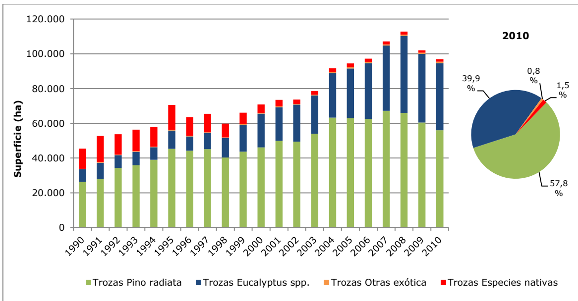
Figura 63. Cosecha: tendencia de la superficie anual por especie, serie 1990-2010
