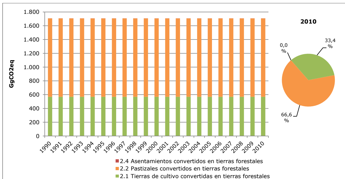
Figura 61. Tierras convertidas en tierras forestales: tendencia de las emisiones de GEI por componente, serie 1990-2010
