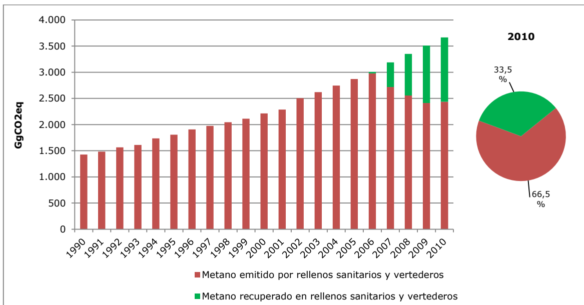
Figura 73. Disposición de residuos sólidos: tendencia del metano emitido y metano recuperado en rellenos sanitarios y vertederos, serie 1990-2010
