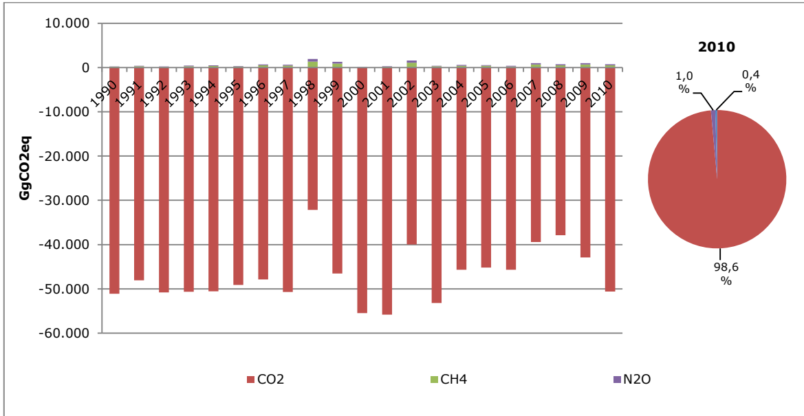
Figura 51. Sector UTCUTS: tendencia de las emisiones y absorciones por tipo de GEI, serie 1990-2010
