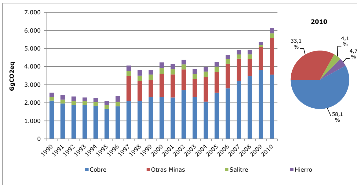
Figura 18. Minería y cantería: tendencia de las emisiones de GEI por componente, serie 1990-2010
