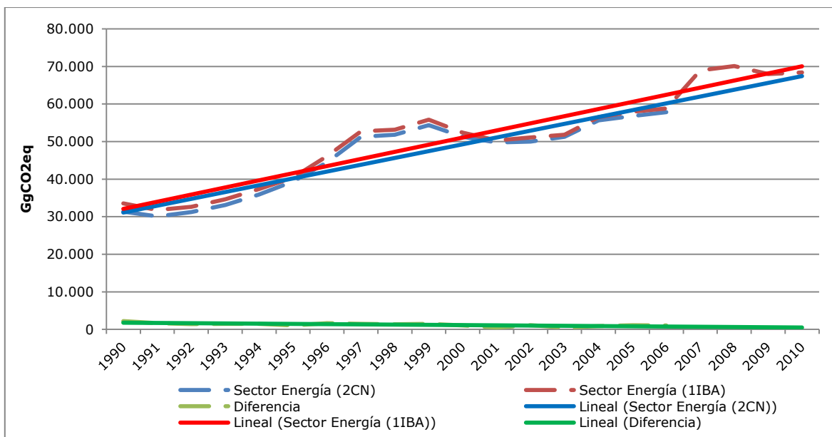
Figura 79. Sector Energía: tendencia de las emisiones de GEI reportadas por Chile en la Segunda Comunicación Nacional y en el Primer Informe Bienal de Actualización, serie 1990-2010
