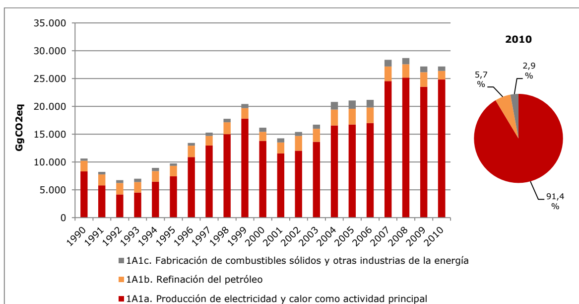
Figura 14. Industria de la energía: tendencia de las emisiones de GEI por componente, serie 1990-2010
