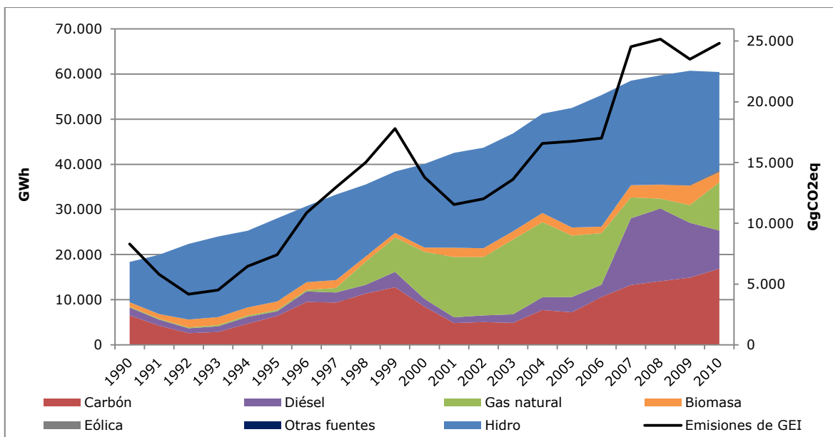
Figura 16. Producción de electricidad y calor como actividad principal: tendencia de la generación eléctrica por tipo de fuente y de las emisiones de GEI, serie 1990-2010
