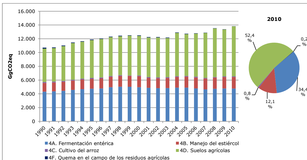
Figura 39. Sector Agricultura: tendencia de las emisiones de GEI por categoría, serie 1990-2010
