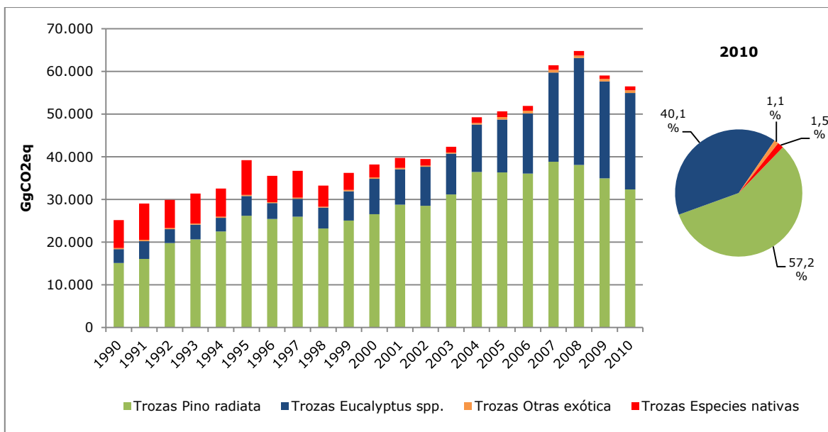
Figura 57. Cosecha: tendencia de las emisiones de CO 2 por especie, serie 1990-2010
