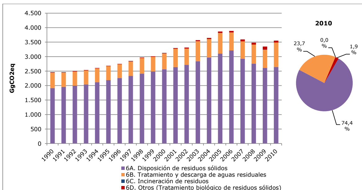
Figura 70. Sector Residuos: tendencia de las emisiones de GEI por categoría, serie 1990-2010
