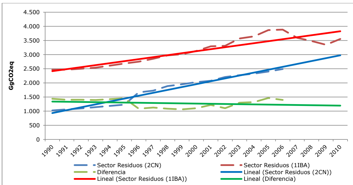
Figura 83. Sector Residuos: tendencia de las emisiones de GEI reportadas por Chile en la Segunda Comunicación Nacional y en el Primer Informe Bienal de Actualización, serie 1990-2010
