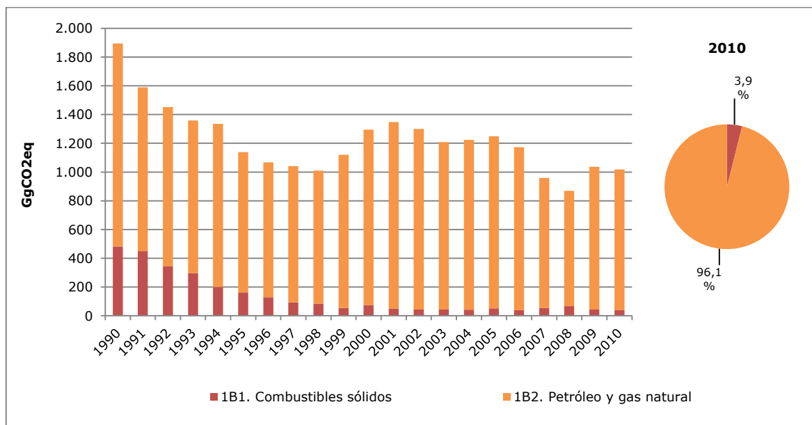
Figura 23. Emisiones fugitivas de combustible: tendencia de las emisiones de GEI por subcategoría, serie 1990-2010
