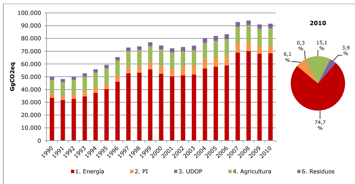
Figura 4. INGEI de Chile: tendencia de las emisiones de GEI por sector (excluyendo UTCUTS), serie 1990-2010
