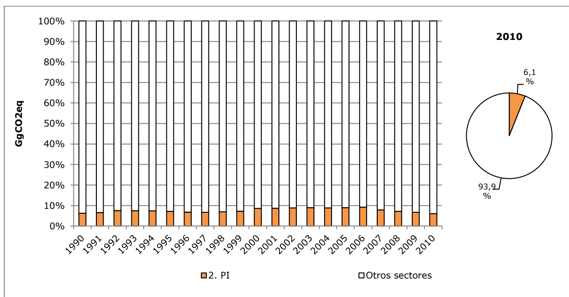
Figura 28. Sector Procesos industriales: tendencia de la participación del sector en las emisiones de GEI totales (excl. UTCUTS)
