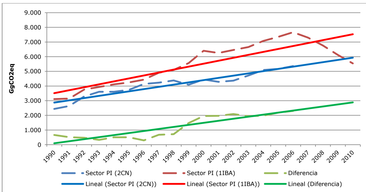
Figura 80. Sector Procesos industriales: tendencia de las emisiones de GEI reportadas por Chile en la Segunda Comunicación Nacional y en el Primer Informe Bienal de Actualización, serie 1990-2010
