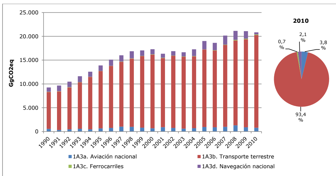
Figura 19. Transporte: tendencia de las emisiones de GEI por componente, serie 1990-2010
