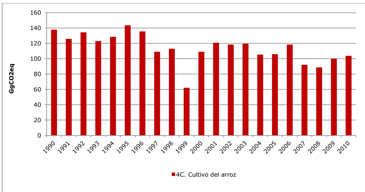
Figura 45. Cultivo del arroz: tendencia de las emisiones de metano, serie 1990-2010
