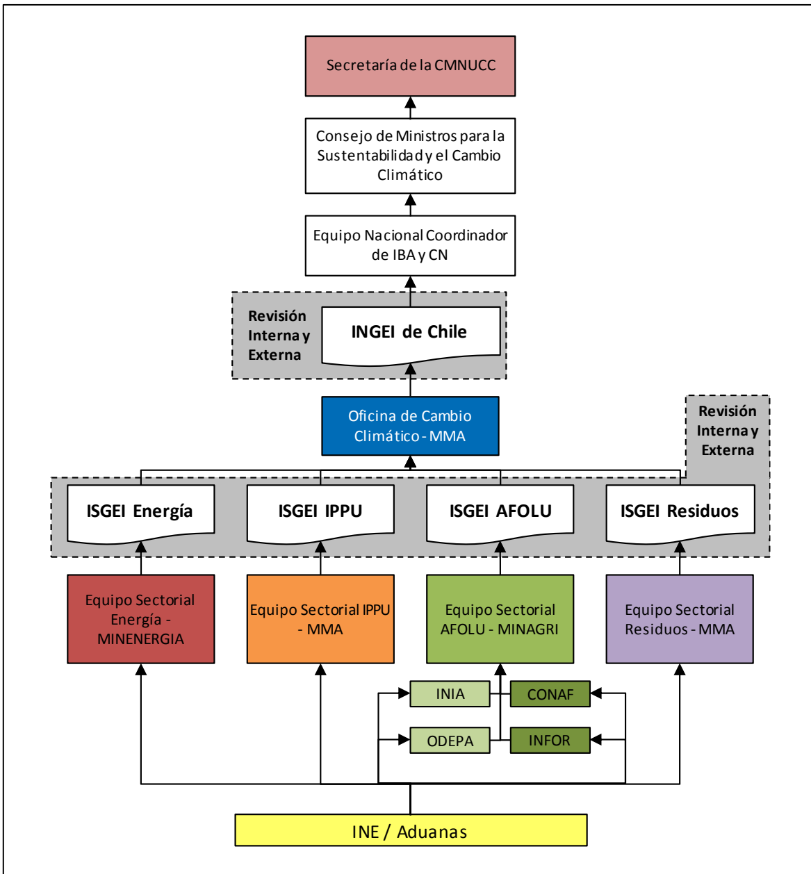
Figura 2. Proceso para la actualización del inventario nacional de gases de efecto invernadero de Chile
