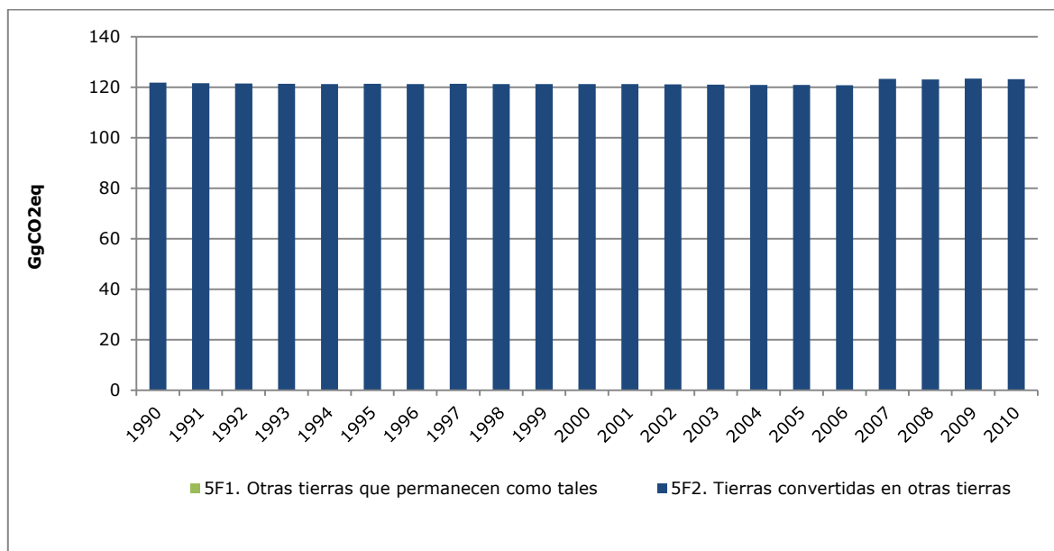
Figura 68. Otras tierras: tendencia de las emisiones y absorciones de GEI por subcategoría, serie 1990-2010
