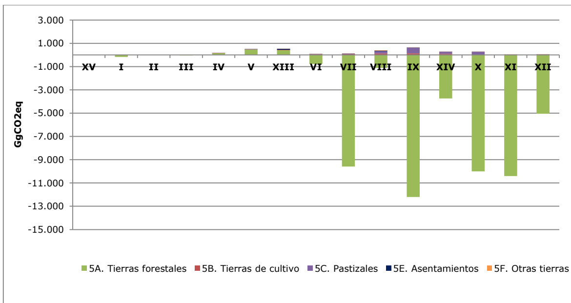
Figura 52. Sector UTCUTS: absorciones y emisiones de GEI por categoría y región administrativa, año 2010
