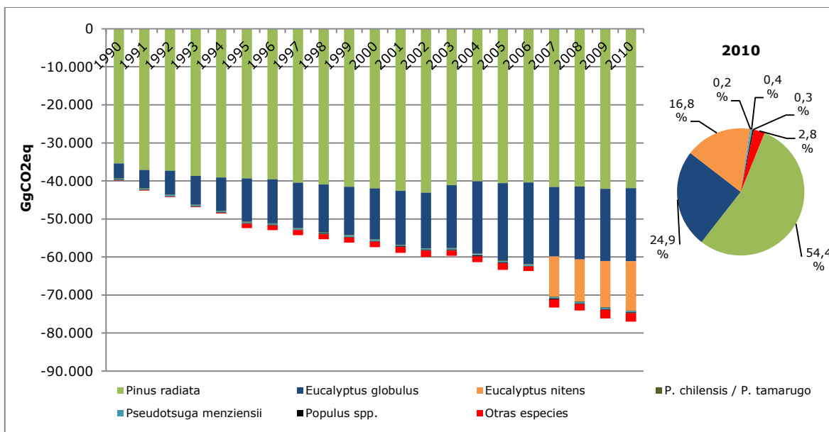
Figura 56. Plantaciones forestales: tendencia de las absorciones de CO 2 por especie, serie 1990-2010
