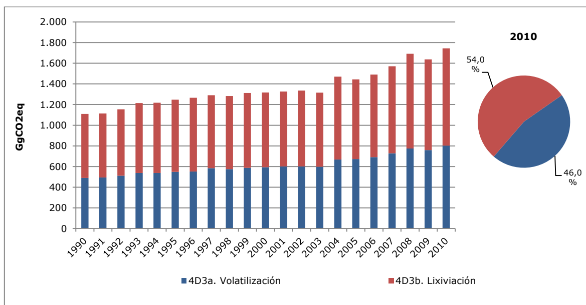
Figura 48. Emisiones indirectas de suelos agrícolas: tendencia de las emisiones de GEI por componente, serie 1990-2010
