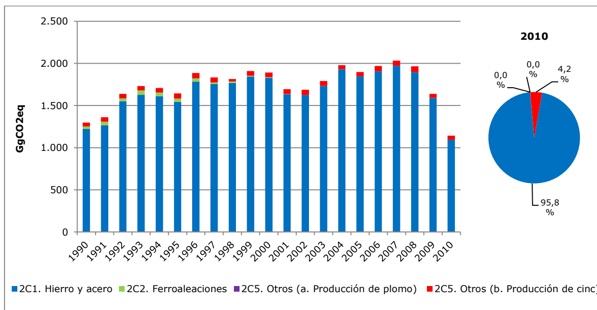
Figura 34. Producción de metales: tendencia de las emisiones de GEI por subcategoría, serie 1990-2010
